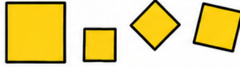
Kare
