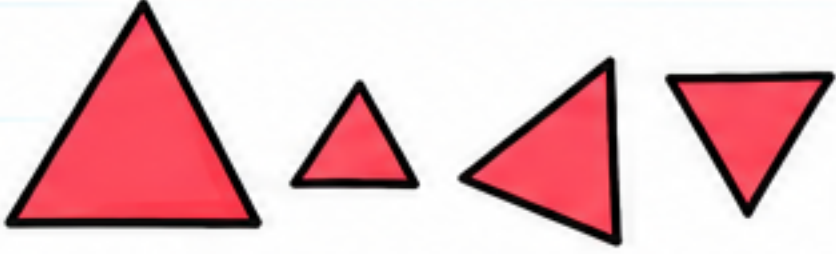
Üçgen
