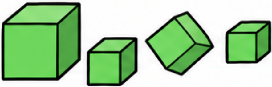
Küp
