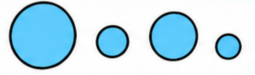
Çember
