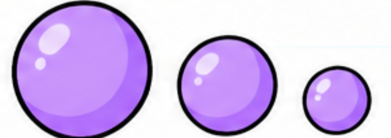
Küre
