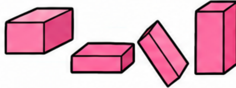
Dikdörtgen prizma
